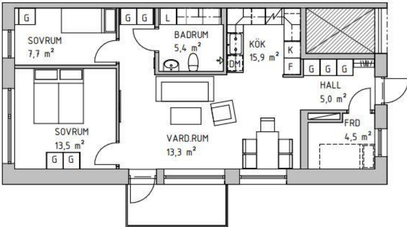
Planskiss
