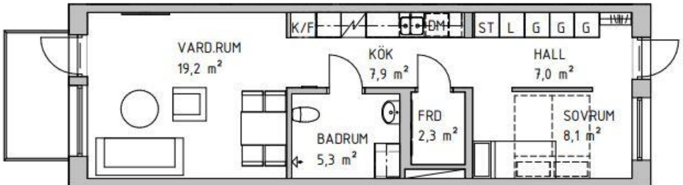
Planskiss
