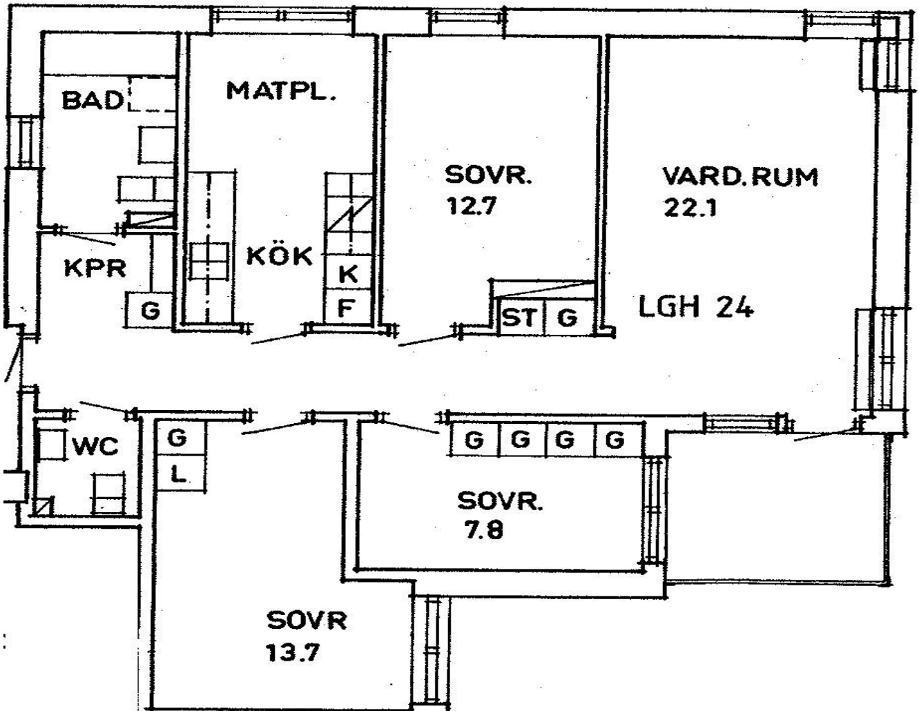
Planskiss
